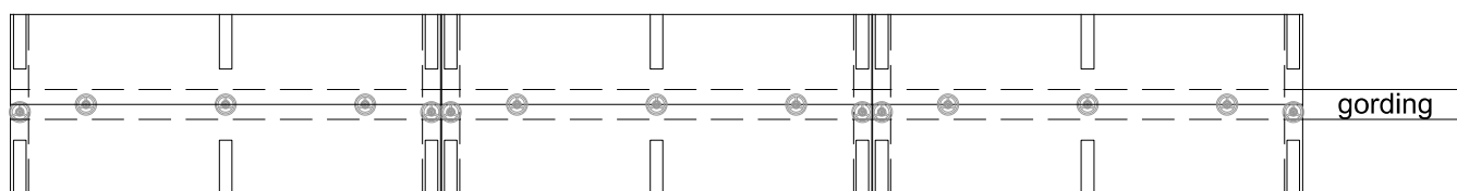
Bevestigingsprincipe t.p.v. stuiknaden bij "SlimFix XT R" dakelementen
