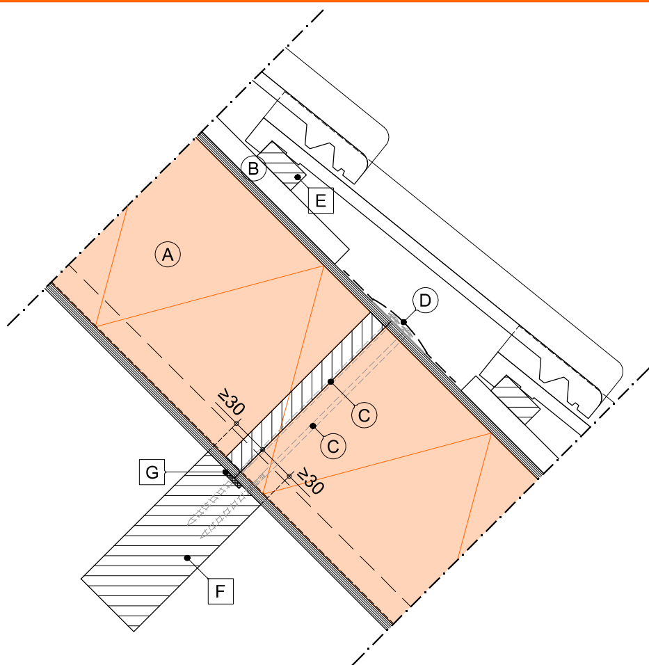
Bevestigingsprincipe t.p.v. stuiknaden bij "SlimFix XT R" dakelementen
